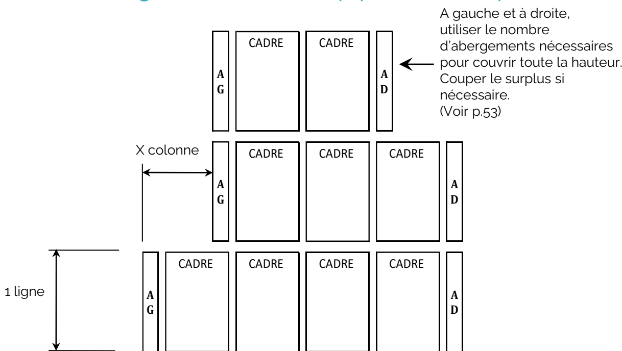
Combinaison multiple pour le dégagement de fenêtre de toit ou de cheminée
