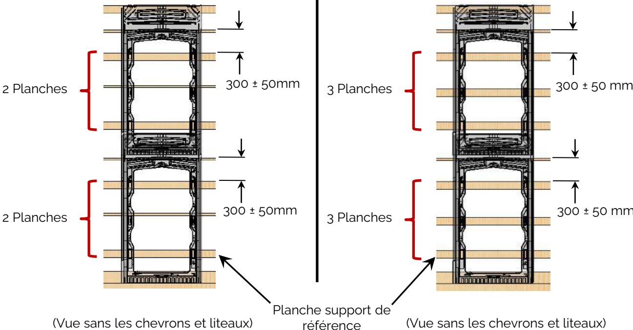
Platelage avec 6 pattes de fixation par panneau PV
