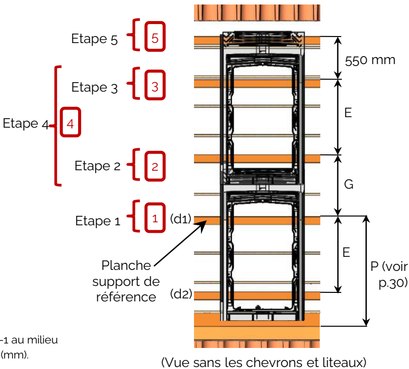
(Vue sans les chevrons et liteaux)
