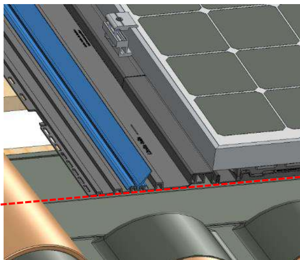
(Bas du champ PV)
