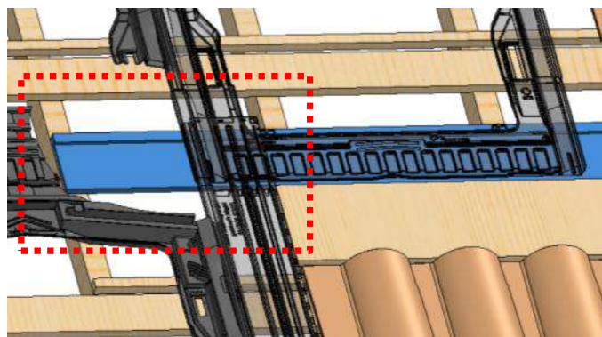
(vue coupe locale des cadres)
