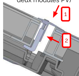
(Vue en coupe entre deux modules PV)
