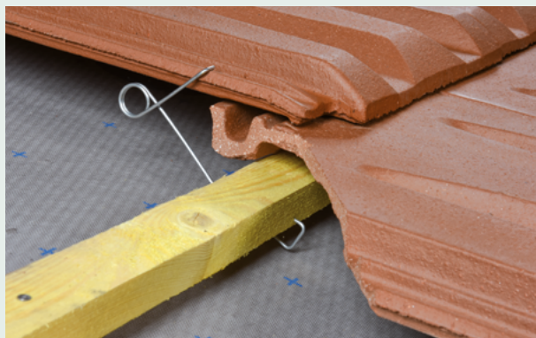
4- Déposer le crochet dans l'emboîtement de la tuile pour assurer la fixation.
