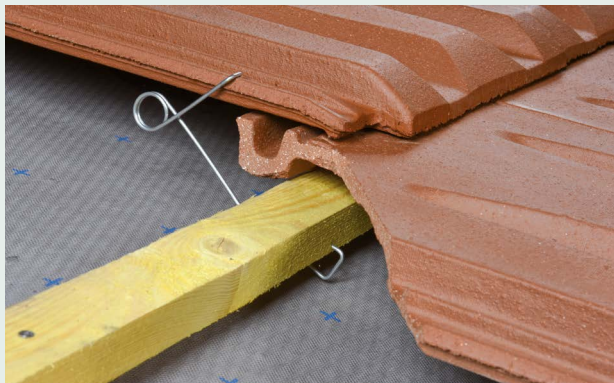
3- Déposer le crochet dans l'emboîtement de la tuile pour assurer la fixation.
