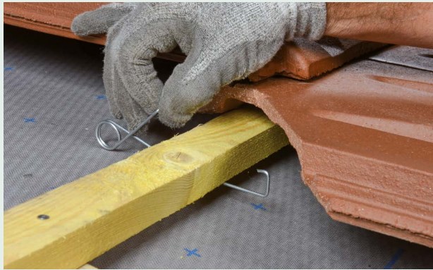
1- Crochet à harponner en sous face du liteau.
