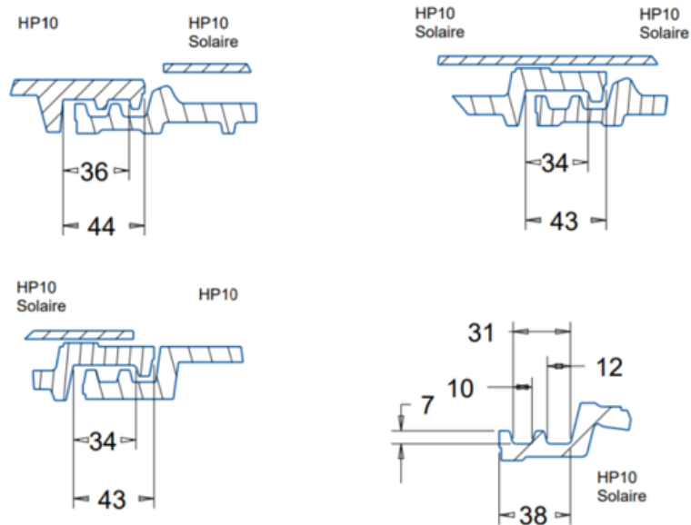
Figure 20 – Emboîtements HP10 Solaire
