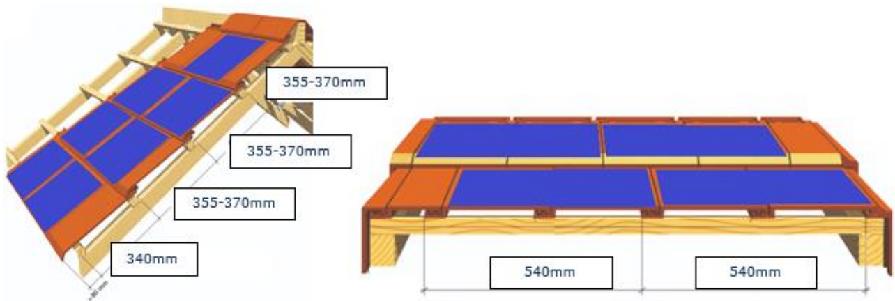
Figure 15 – Pureaux / Largeurs utiles Alpha Solaire
