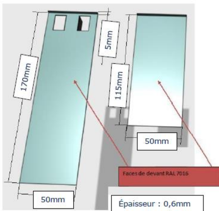
Figure 8 – Cache de protection Câbles Solaires
