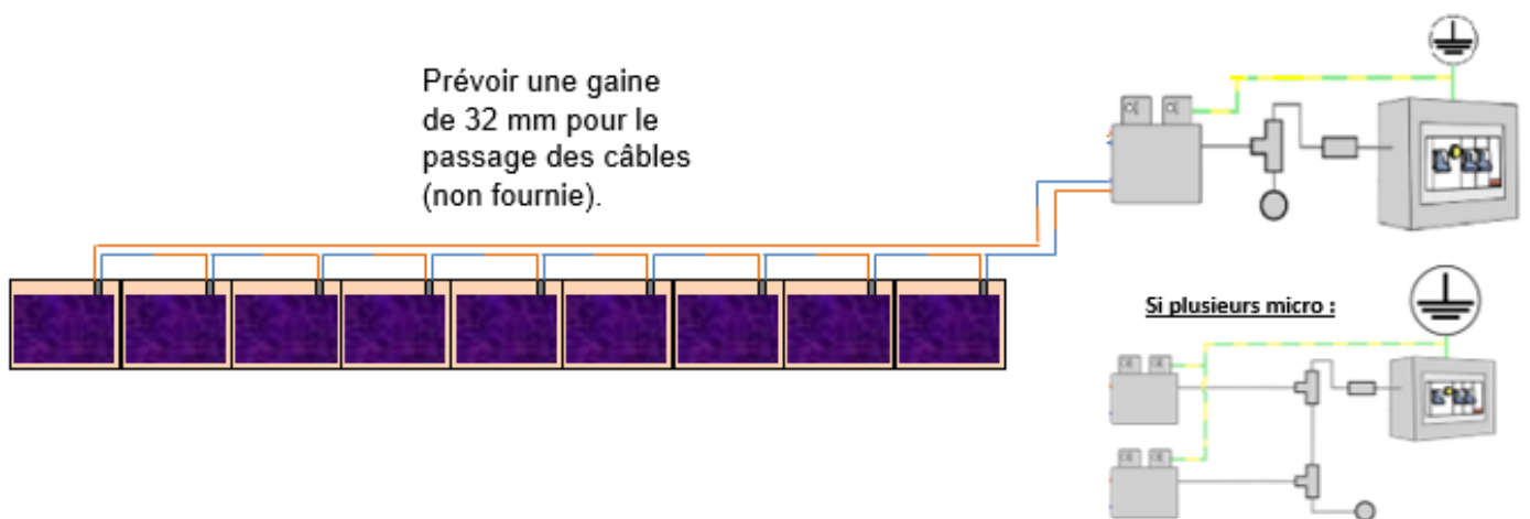
Figure 11 – Principe de câblage électrique sur micro onduleur
