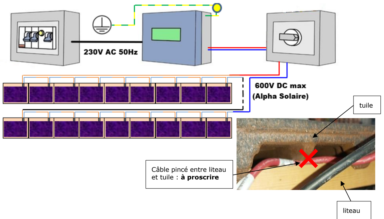
Figure 10 – Principe de câblage électrique sur onduleur décentralisé
