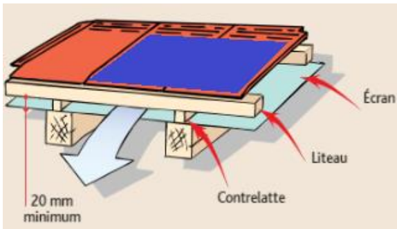
Figure 12 – Pose avec écran de sous toiture
