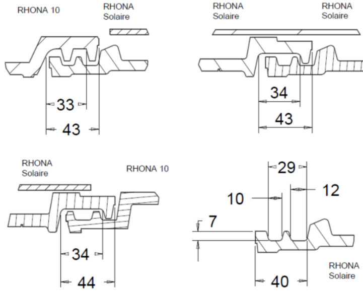
Figure 19 – Emboîtements Rhôna Solaire
