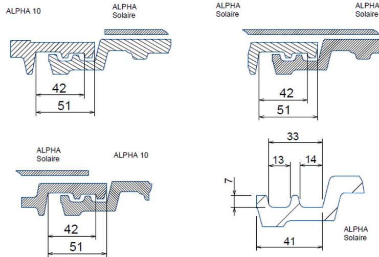
Figure 18 – Emboîtements Alpha Solaire
