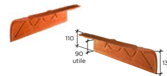
Rive ronde individuelle à emboîtement (2,6 par ml au pureau de 392 mm) Gauche Réf. 106.55 Droite Réf. 106.56
