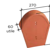
Fronton 90° modèle pour faitière à pureau variable à emboîtement (grande ouverture) et rabat 90° Réf. 814
