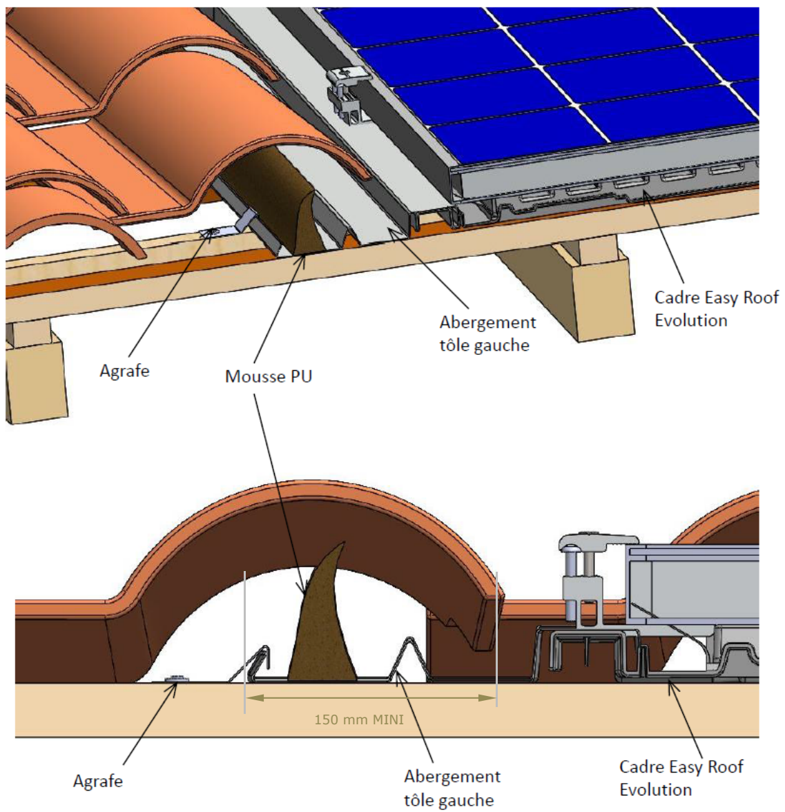
Figure 41 – Mise en place des éléments de couverture sur les abergements latéraux métalliques
