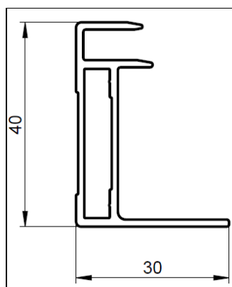
Figure 10 – Cadre du module photovoltaïque SolarWatt
