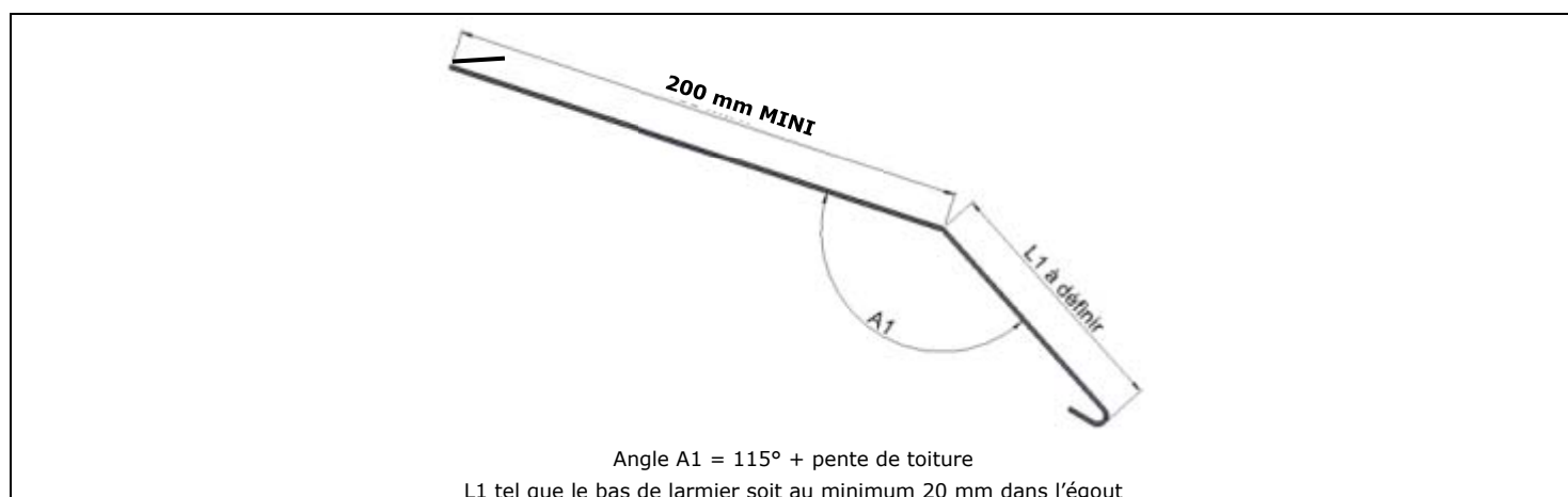
Figure 21 – Larmier pour raccordement à l'égout
