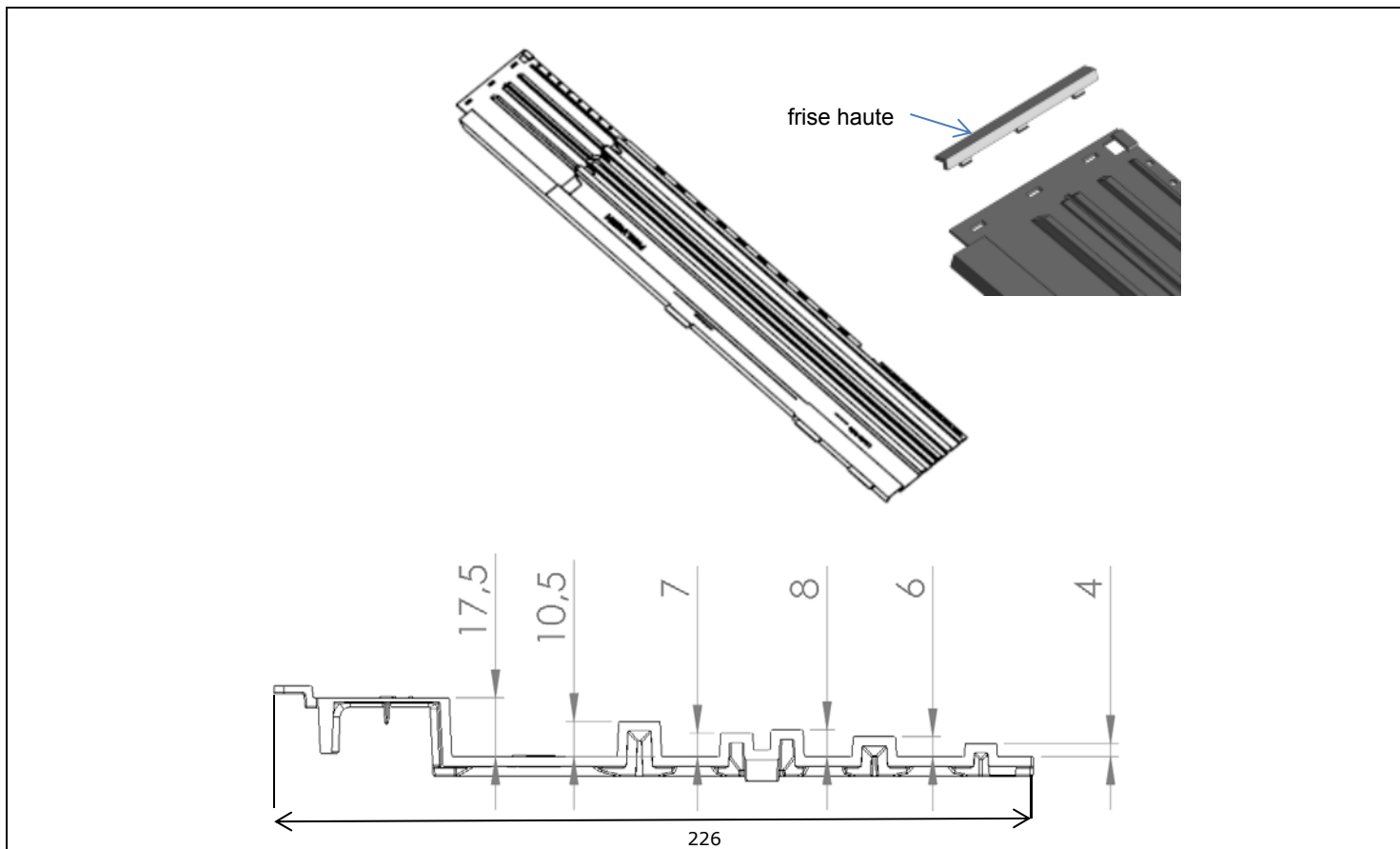
Figure 17 – Abergement latéral droit
