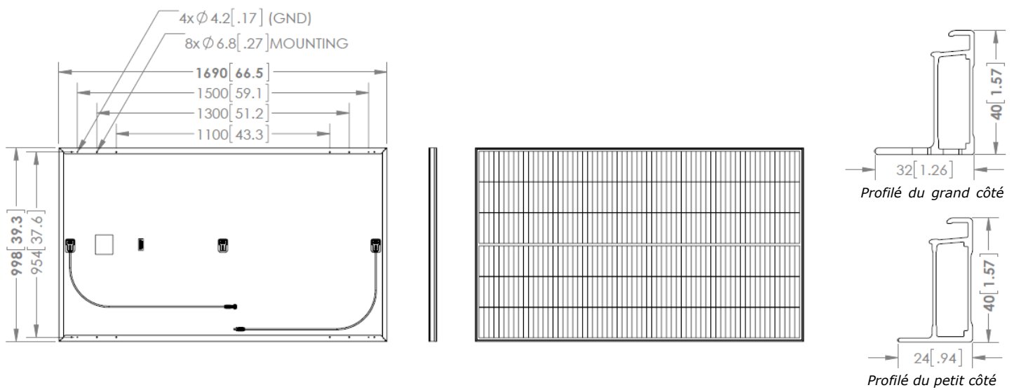
Figure 8 – Modules photovoltaïques SunPower SPR-P19-xxx-BLK et son cadre
