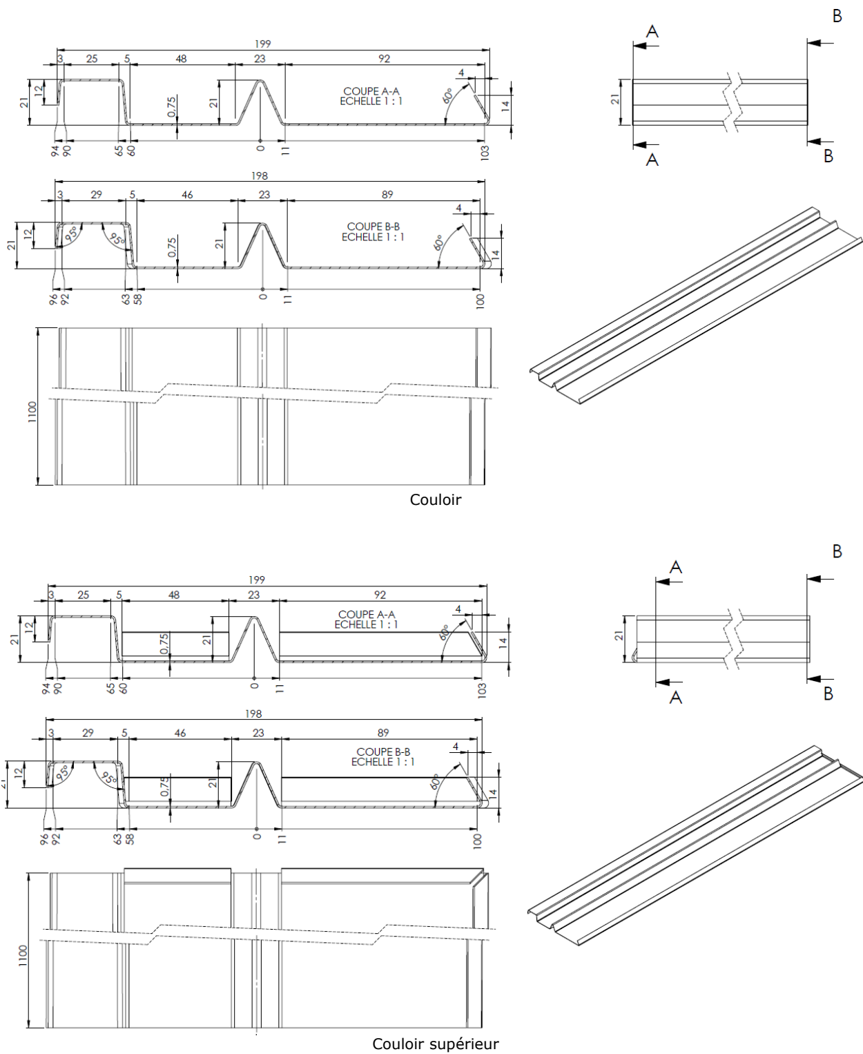
Figure 23 – Abergement latéral métallique (exemple : couloir droit)
