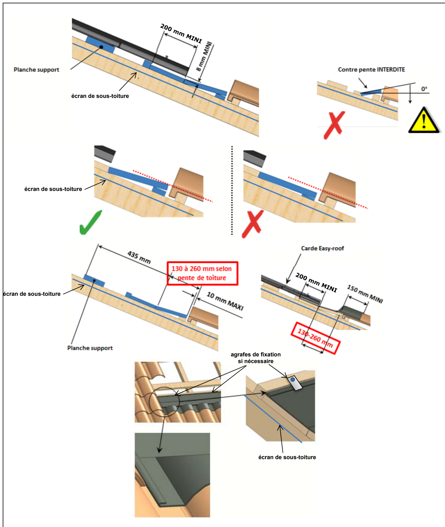
Figure 29 – Pose du bas de champ
