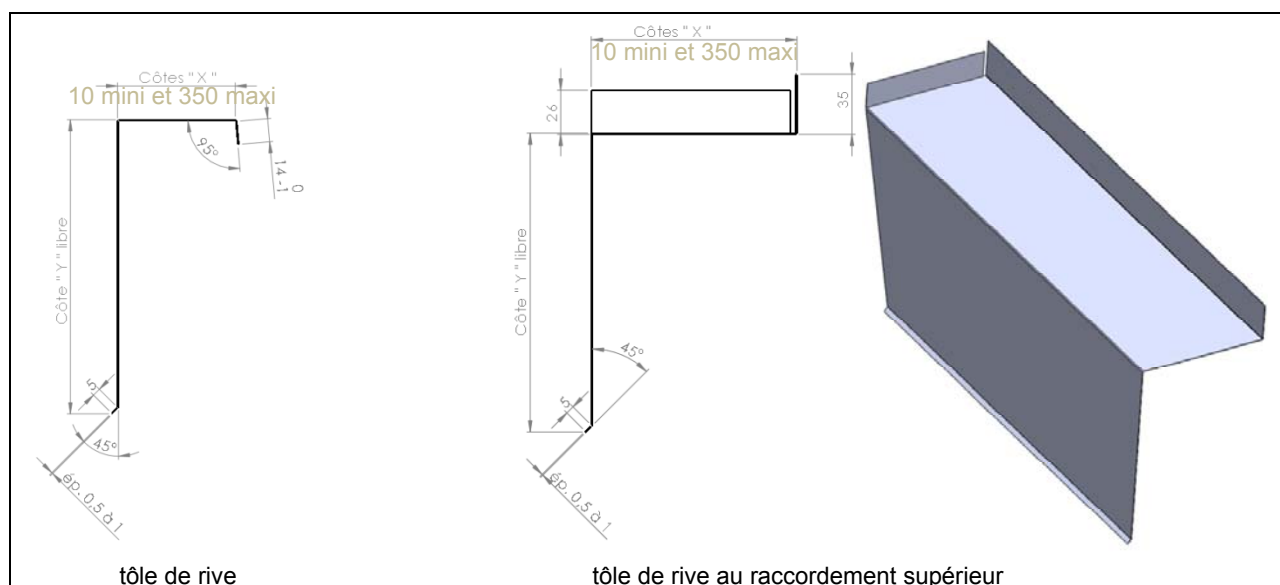
Figure 22 – Abergement de rive latérale
