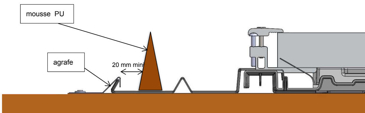
Figure 35 – Pose des abergements latéraux métalliques
