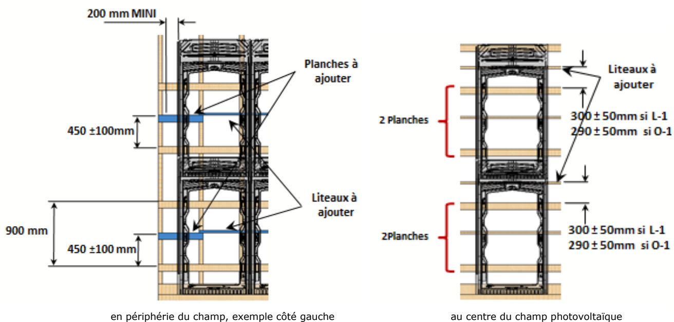
Figure 30 – Platelage du champ photovoltaïque avec 4 pattes de fixation par module
