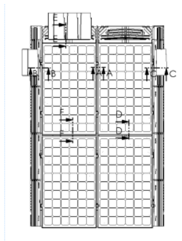
Figure 36 – Vue en coupe longitudinale du procédé en partie courante
