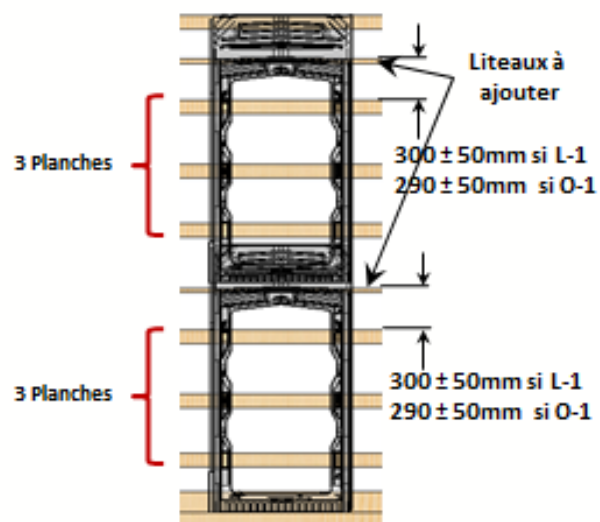
Figure 31 – Platelage du champ photovoltaïque avec 6 pattes de fixation par module
