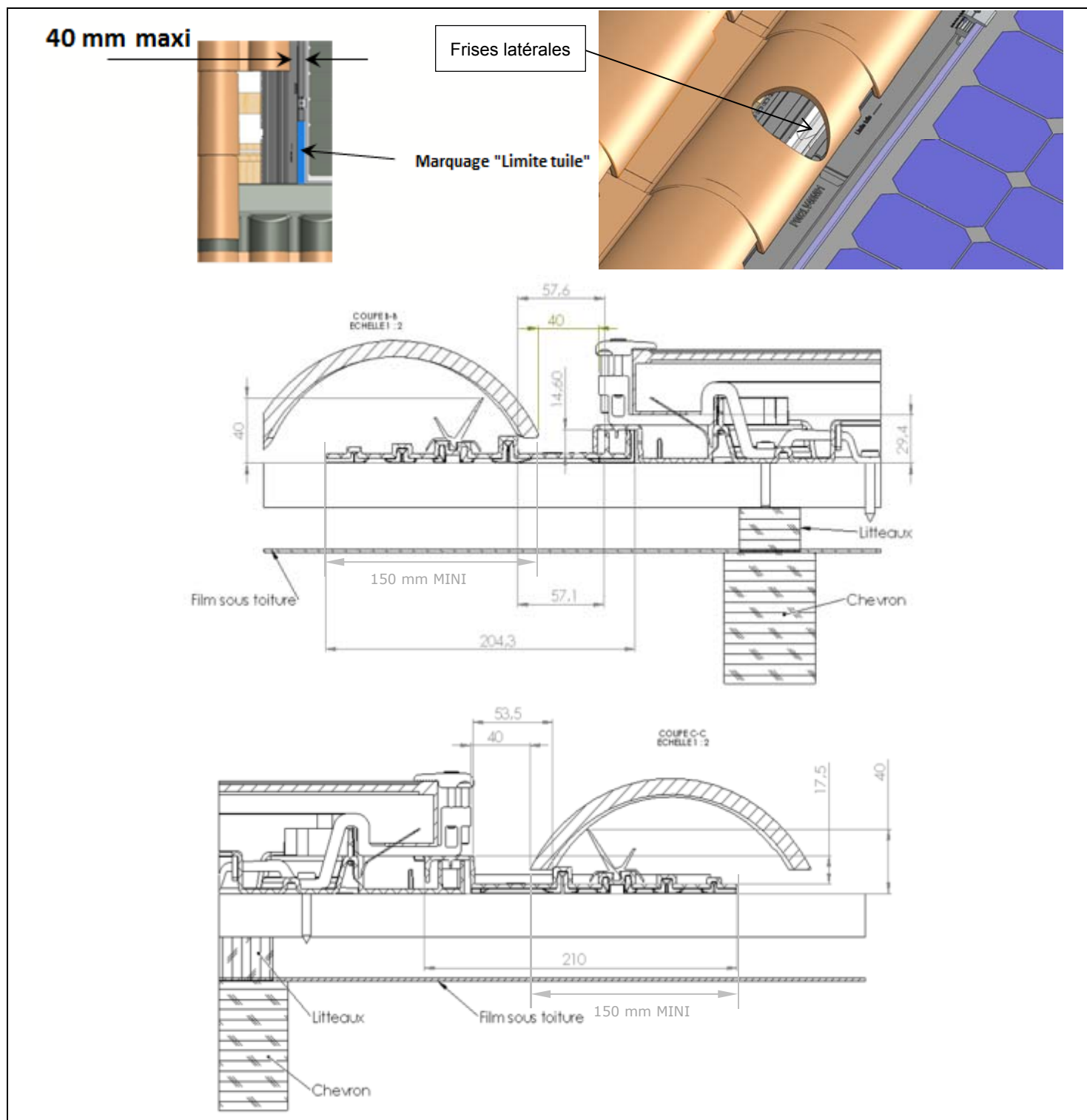
Figure 40 – Mise en place des éléments de couverture sur les abergements latéraux polymère
