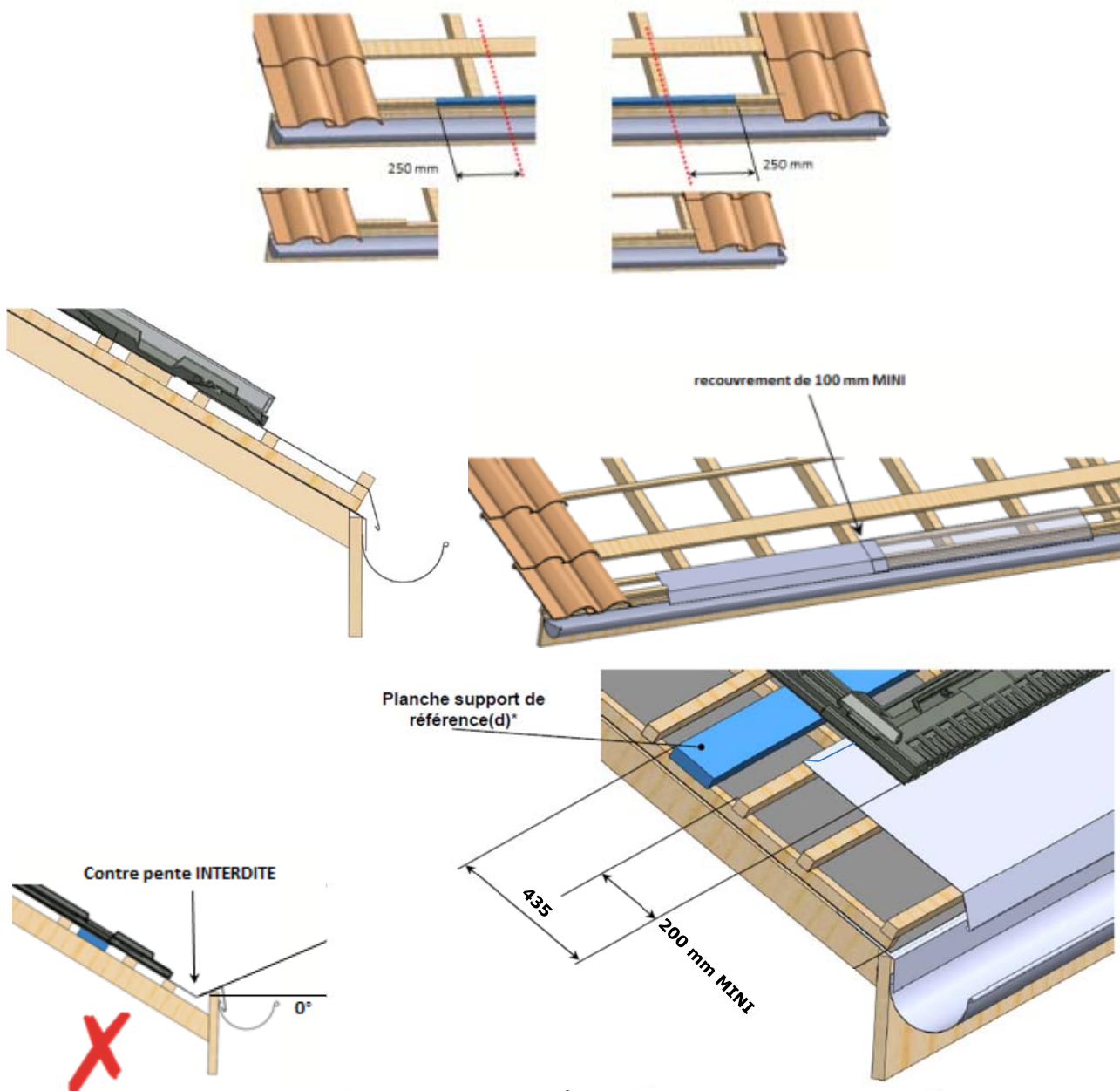
Figure 42 – Pose à l'égout
