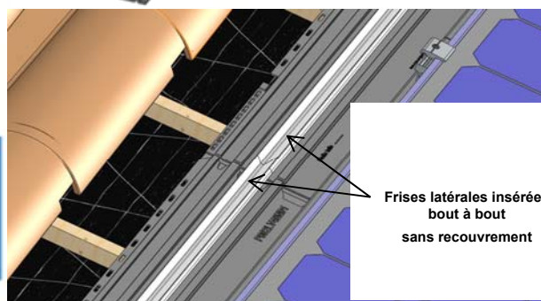
Figure 34 – Pose des abergements latéraux
