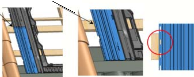
Figure 34 – Pose des abergements latéraux
