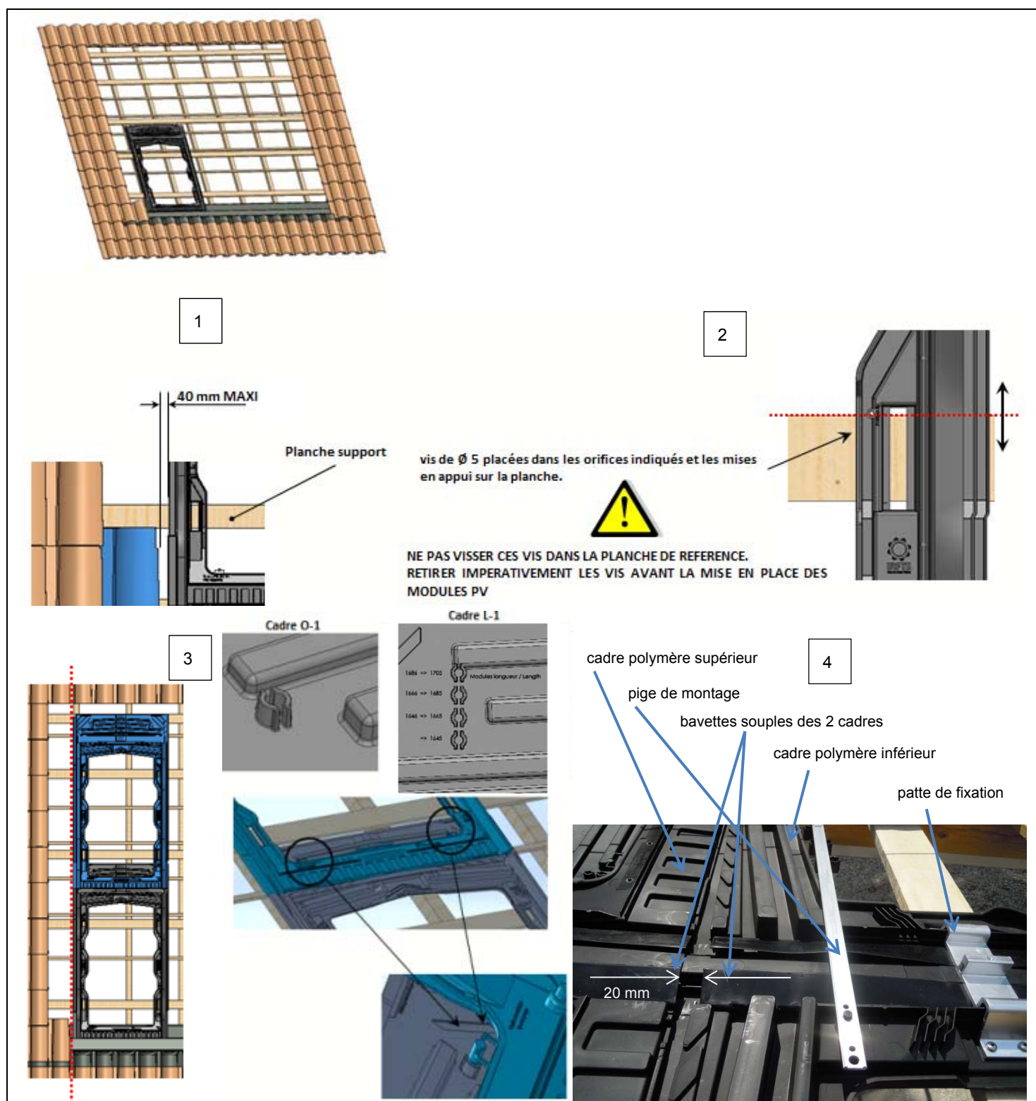
Figure 32 – Pose des cadres Easy-Roof
