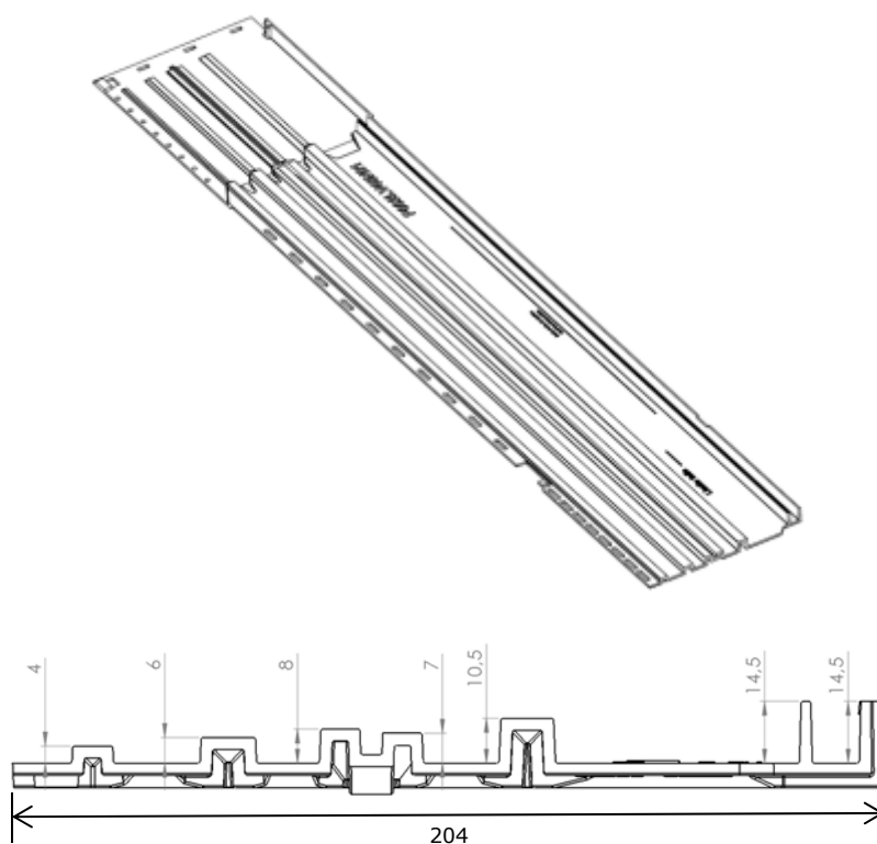
Figure 16 – Abergement latéral gauche
