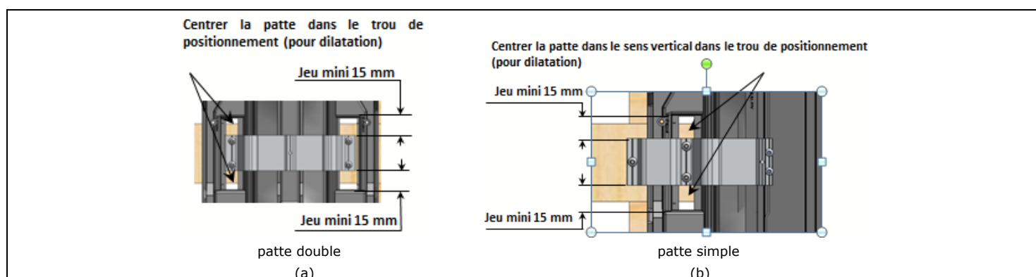
Figure 33 – Fixation des pattes
