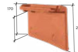
Rive individuelle VALOISE Huguenot (3,8 au ml) Droite à emboîtement Réf. 310.43
