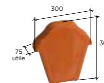
Fronton pour faîtière ondulée à emboîtement Réf. 810
